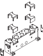
placa de entrada 26 mm alimentação externa do piloto
