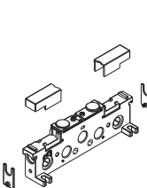
placa de entrada 14,5 mm alimentação externa do piloto
