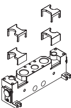
placa de entrada 26 mm alimentação interna do piloto
