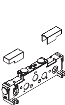
placa de entrada 14,5 mm alimentação interna do piloto
